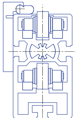
BS100 Staurollenkette 3/4"/ Roller chain 3/4"/ Convoyeur d'accumulation à rouleaux 3/4"
