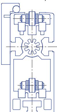
BS11 Staurollenkette 1/2"/ Roller chain 1/2"/ Convoyeur d'accumulation à rouleaux 1/2"
