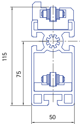
BS10 Staurollenkette/ Roller chain/ Convoyeur d'accumulation à rouleaux 1/2"
